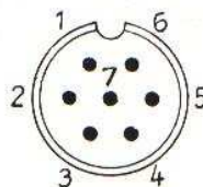
Kontakte der Steckereinsätze – Ansichten Lötseite Doseneinsätze spiegelbildlich
