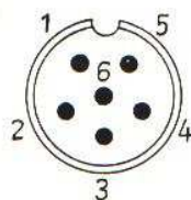
Kontakte der Steckereinsätze – Ansichten Lötseite Doseneinsätze spiegelbildlich
