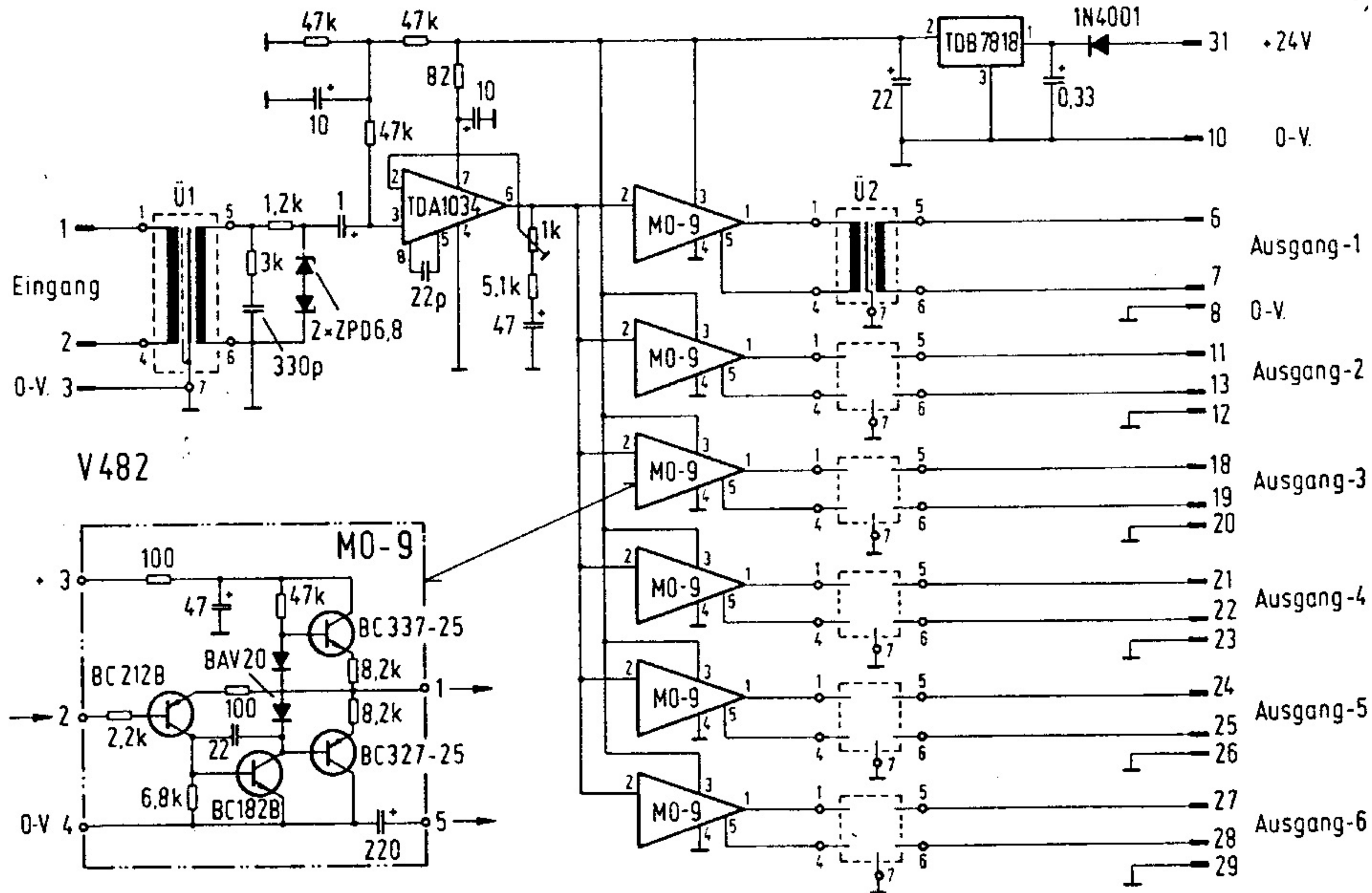
Bild E 66. Verteiler-Verstärker V482 (Neumann)
